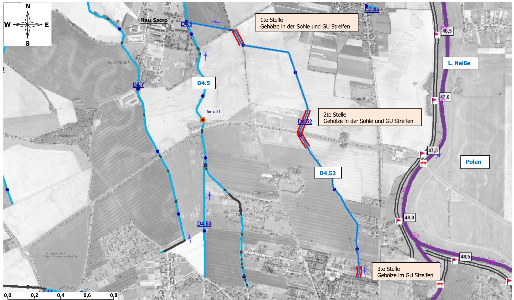
Gehölzplan Blatt D4.52 Graben 86 Forst Neu Sacro Astwerk im QS + GU-Streifen einseitig
